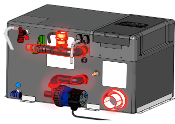
Värmepanna Alde Compact 3030/3030 Plus
