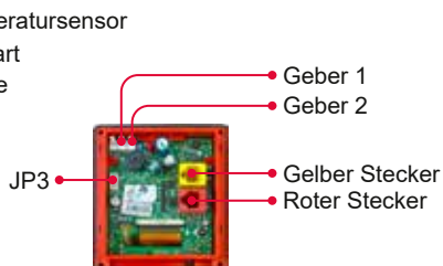
Abb. 21. Anschlüsse am Bedienteil
